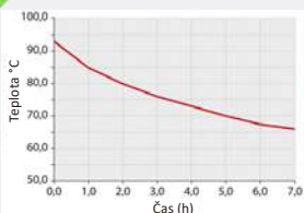
Teplotná krivka pri 20°C okolitej teplote
